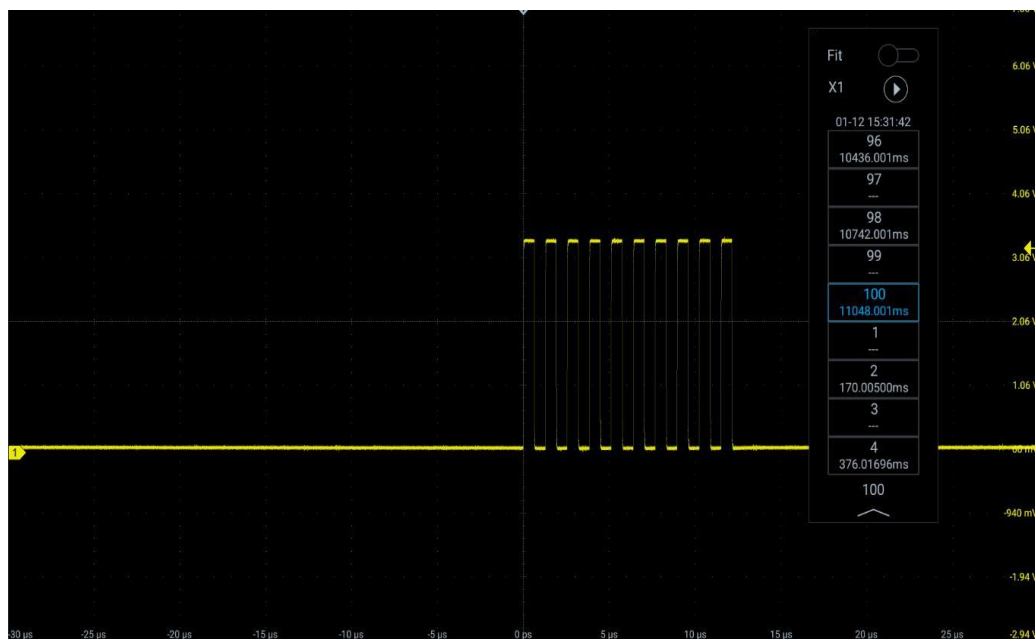
Рисунок 10-13. Сегментированное хранение с просмотром одного кадра
