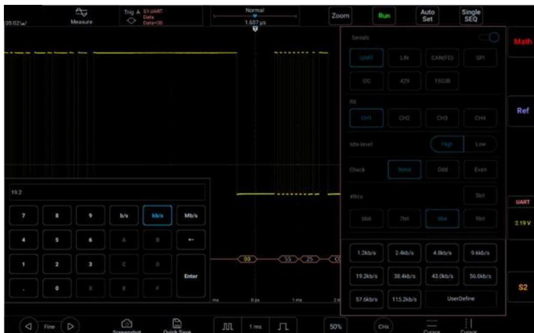
Рисунок 11-5. Настройка скорости передачи данных по умолчанию
