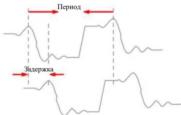
Рисунок 6-6. Схема измерения фазы
