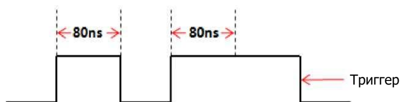
Рисунок 5-17. Время триггера T > 80 нс
