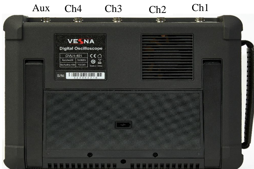
Рисунок 2-3. Задняя панель
