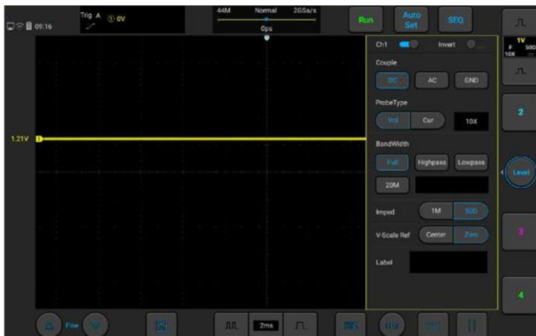
Рисунок 4-17. Входное полное сопротивление канала
