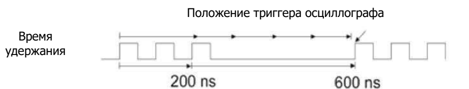
Рисунок 6-10. Время удержания триггера
