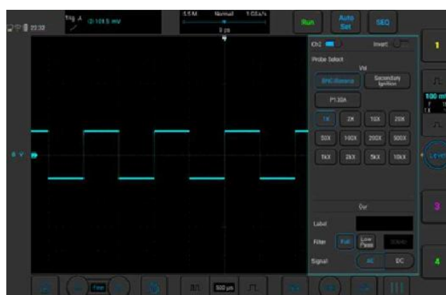
Рисунок 5-8. Связь по переменному току
