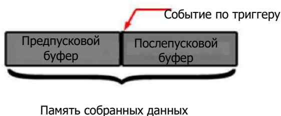
Рисунок 6-6. Концептуальная демонстрация памяти собранных данных
