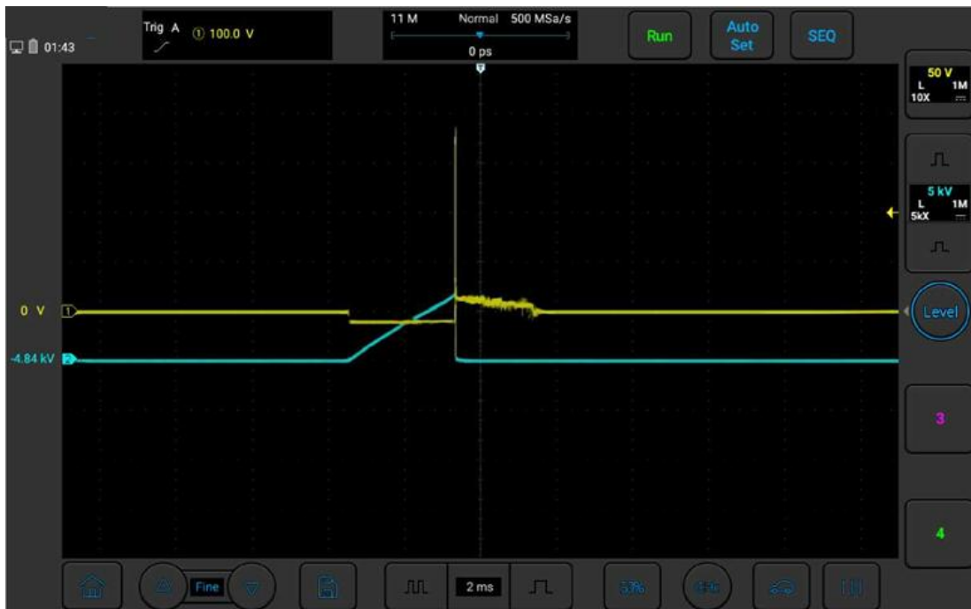
Рисунок 3-45. Первичный + вторичный сигнал зажигания двигателя BMW 5 серии N20
