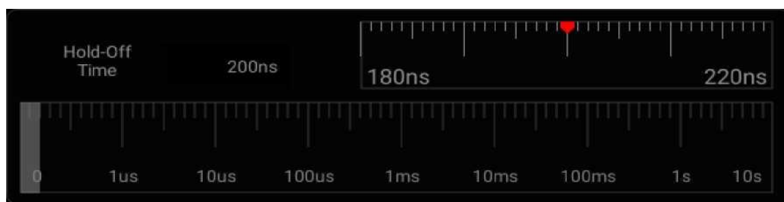
Рисунок 6-11. Интерфейс установки времени удержания триггера
