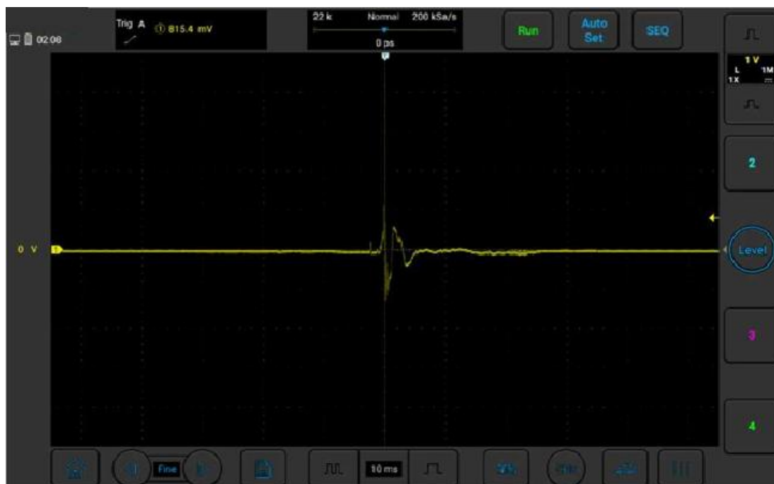
Рисунок 3-20. Измерения датчика детонации
