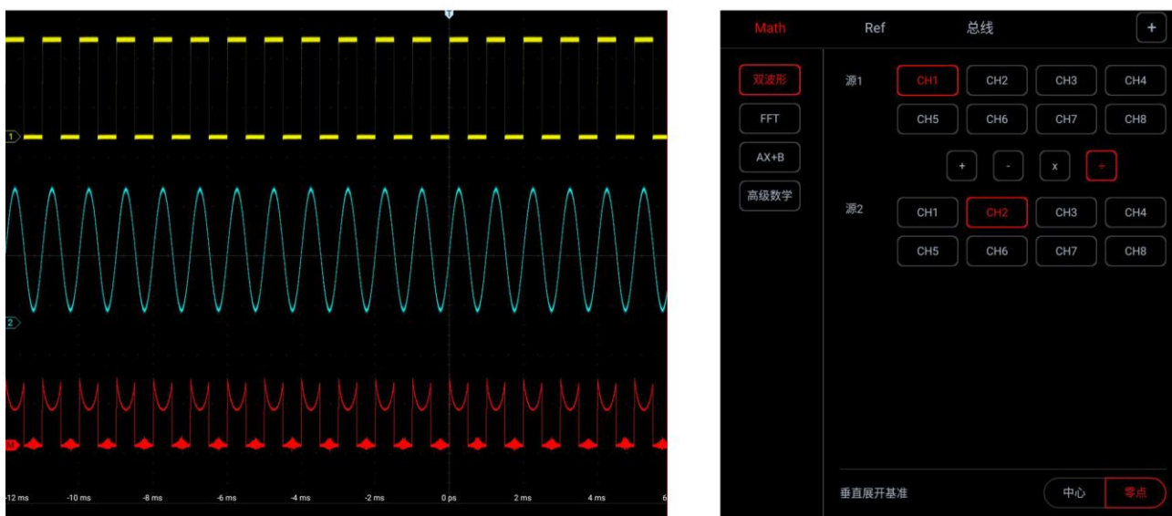
Рисунок 9-1. Форма сигнала математического канала
