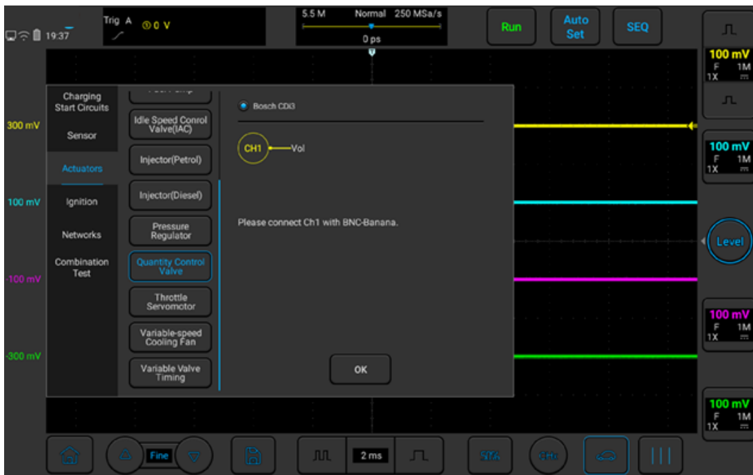
Рисунок 3-35. Проверка клапана управления количеством (расходом)
