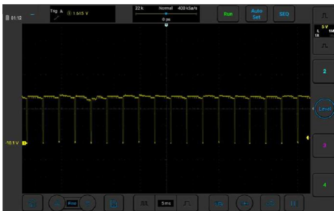
Рисунок 3-39. Проверка изменения фаз газораспределения
