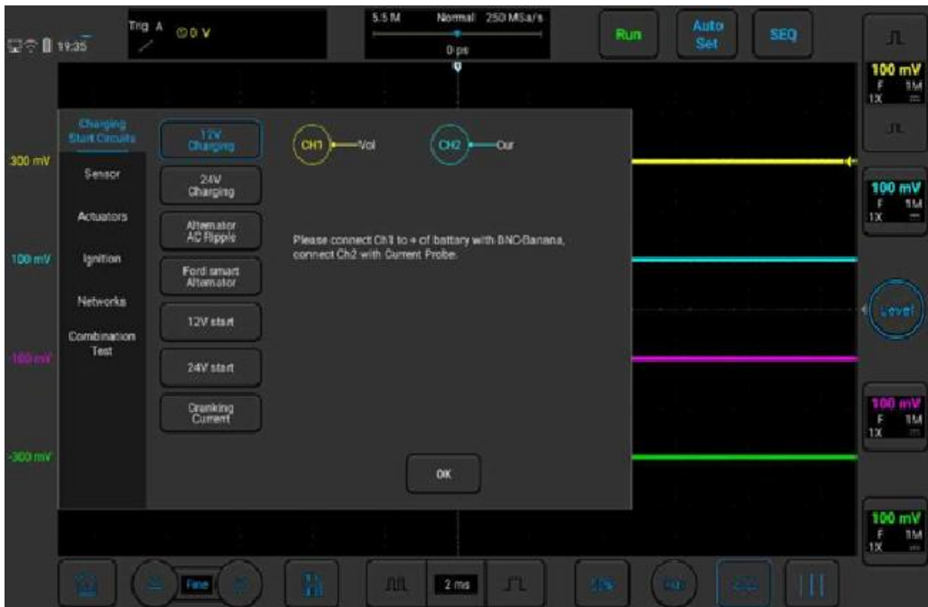
Рисунок 3-2. Зарядка 12 В
