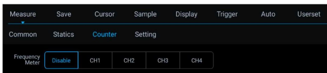
Рисунок 7-9. Открытие меню измерений частотомера
