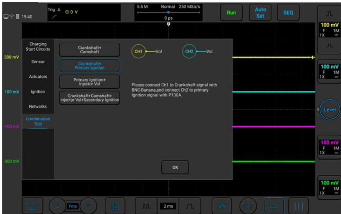
Рисунок 3-51. Комбинированное испытание коленчатого вала и первичной обмотки системы зажигания
