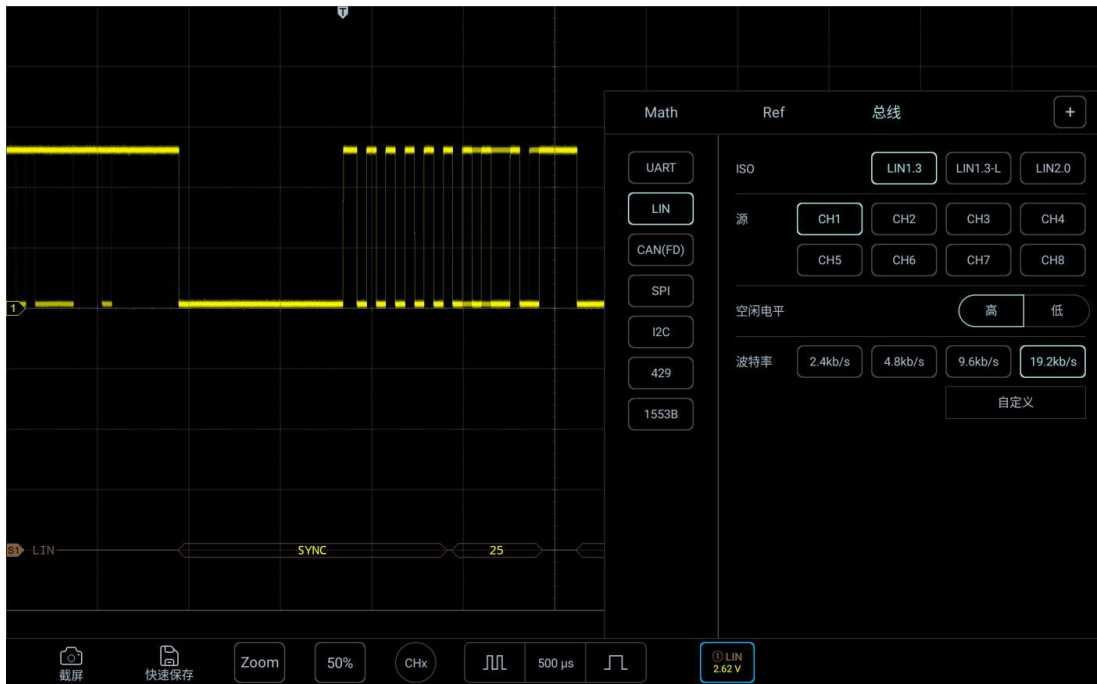
Рисунок 12-10. Меню конфигурации шины LIN
