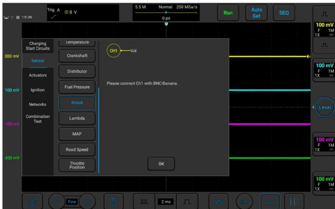
Рисунок 3-19. Тест датчика детонации
