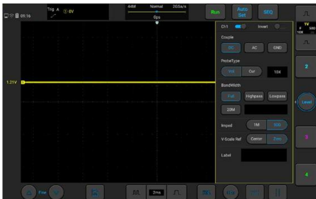
Рисунок 5-14. Входное полное сопротивление канала
