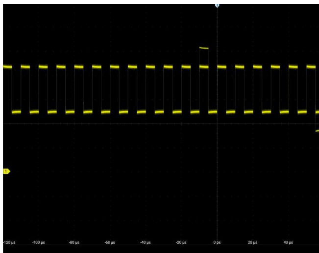
Рисунок 6-3. Аномальный сигнал в периодических сигналах
