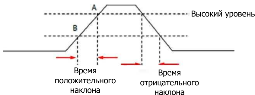
Рисунок 7-26. Время положительного/отрицательного наклона
