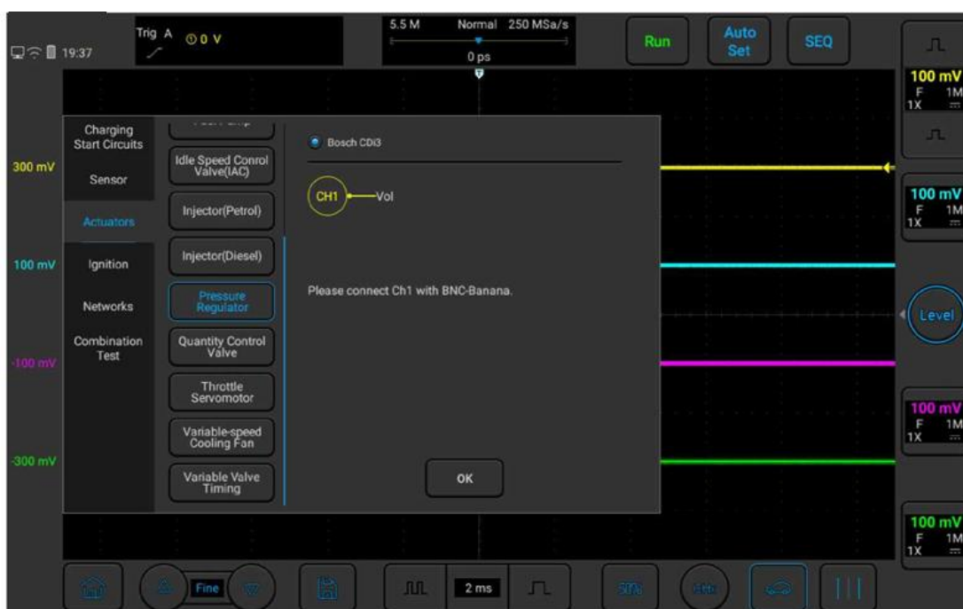
Рисунок 4-9. Проверка регулятора давления
