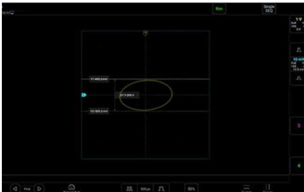
Рисунок 5-26. Измерение разности фаз и использование курсора
