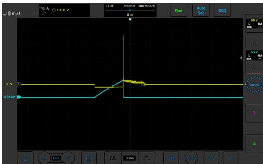
Рисунок 5-5. Первичный + вторичный сигнал зажигания двигателя BMW 5 серии N20
