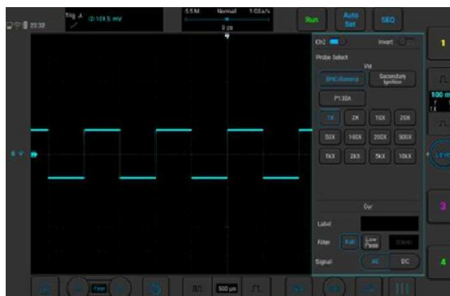
Рисунок 5-35. Связь по переменному току
