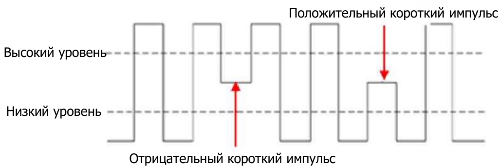
Рисунок 7-24. Короткий триггер
