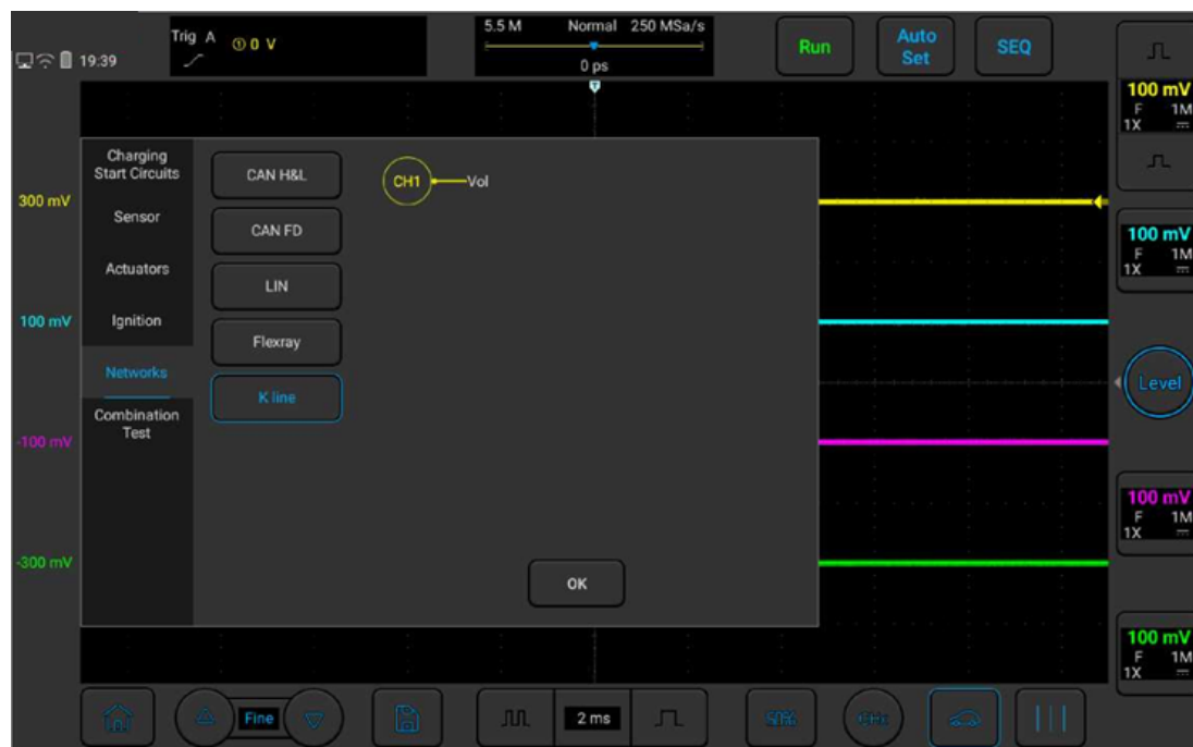
Рисунок 5-10. Проверка K-линии
