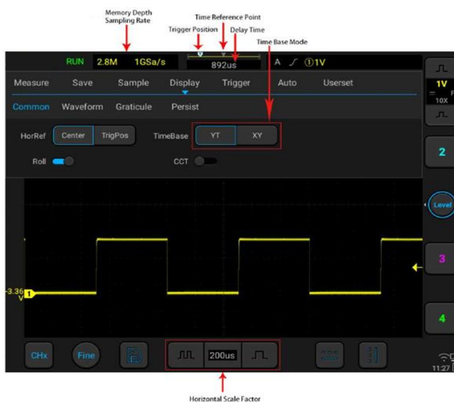
Рисунок 5-17. Горизонтальная система
