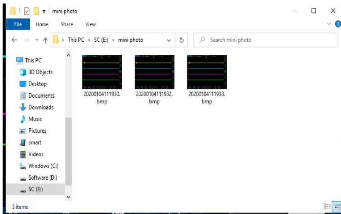
Рисунок 14-5. Просмотр изображений
