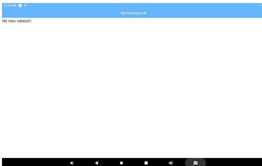
Рисунок 15-1. Приложение SystemUpgrade
