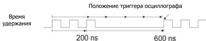
Рисунок 6-10. Время удержания триггера
