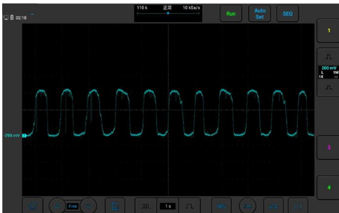
Рисунок 3-21. Диаграмма лямбда-датчика (датчика кислорода)
