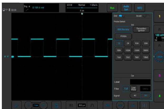
Рисунок 5-34. Связь по постоянному току
