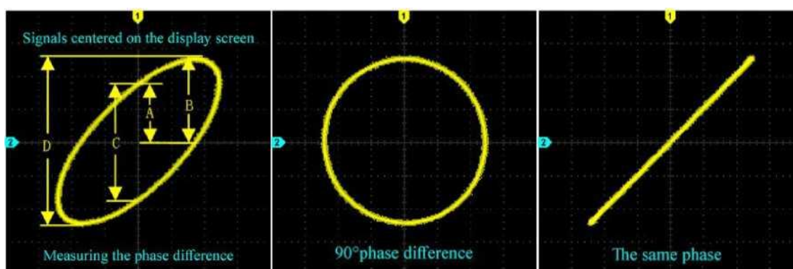
Рисунок 5-25. Сигнал режима строчной развертки «XY», центр экрана дисплея
