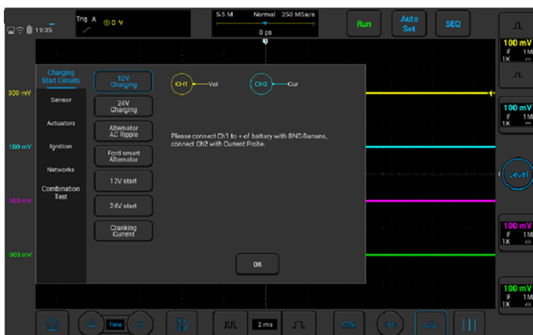
Рисунок 3-1. Цепи зарядки/пуска
