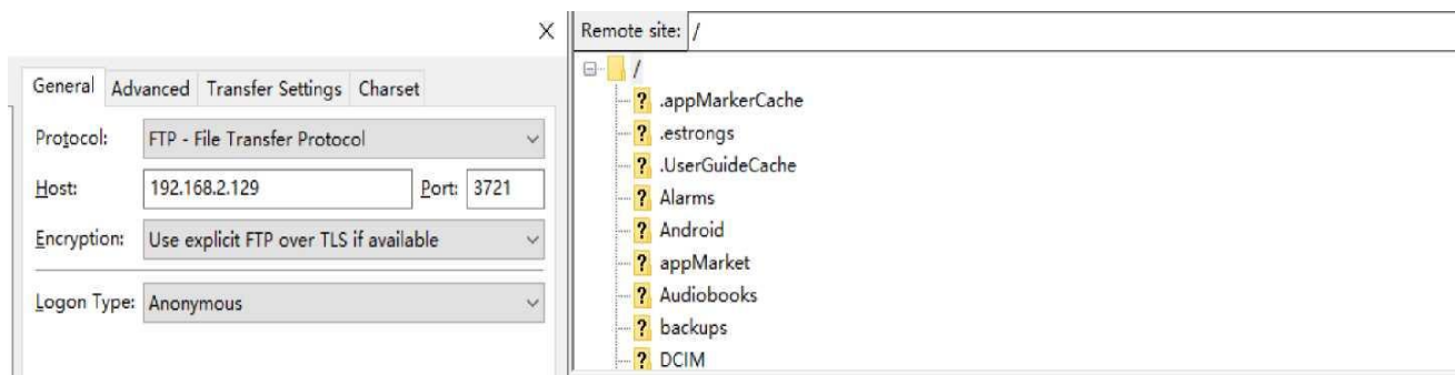
Рисунок 13-15. FileZilla
