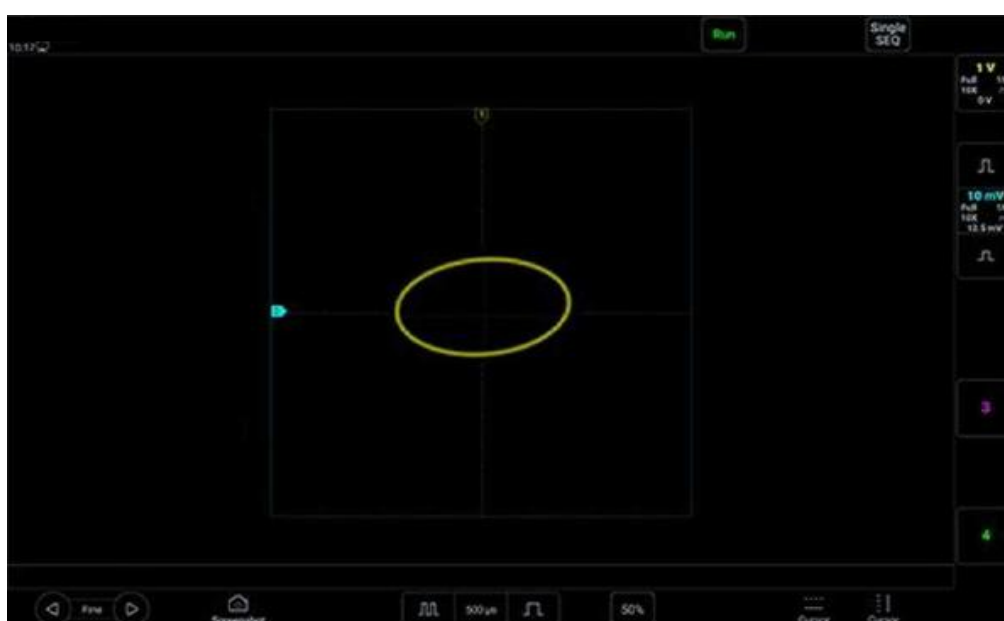
Рисунок 5-24. Режим «XY»
