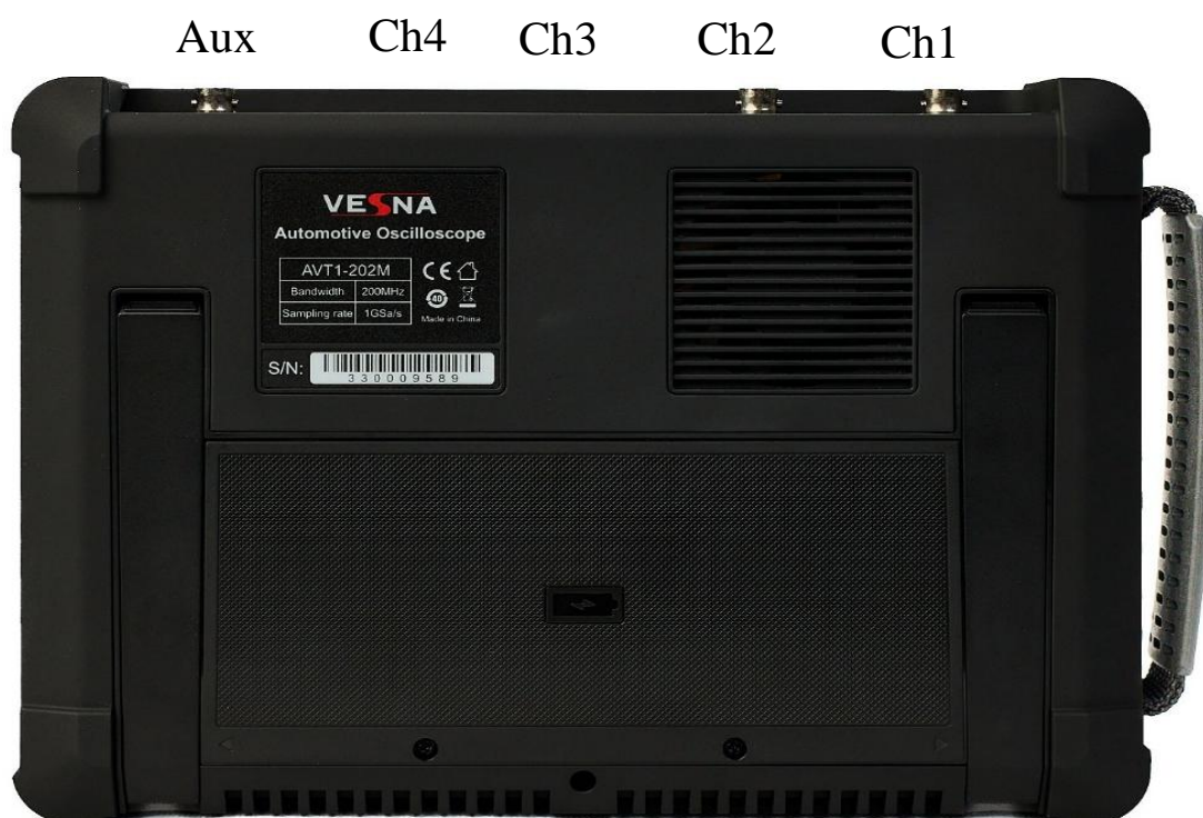
Рисунок 2-3. Задняя панель
