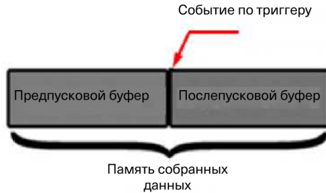
Рисунок 6-6. Концептуальная демонстрация памяти собранных данных
