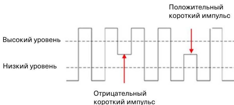
Рисунок 6-24. Кроткий триггер
