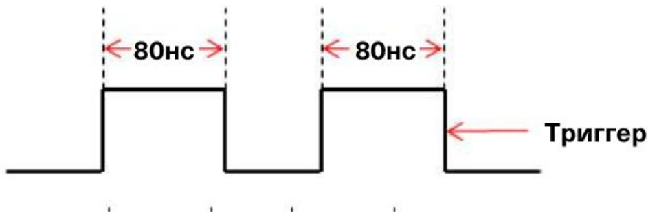
Рисунок 6-18. Время триггера T = 80 нс
