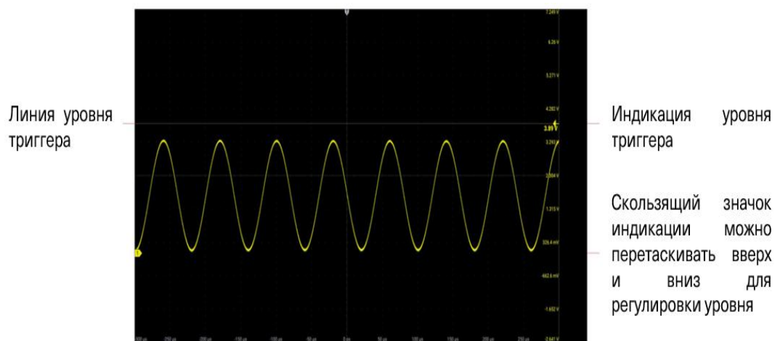
Рисунок 6-8. Уровень триггера
