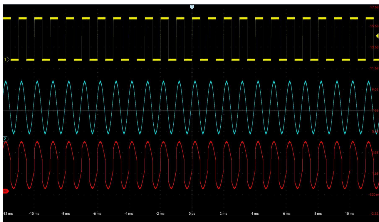
Рисунок 9-2. Математическая операция сложения CH1 и CH2
