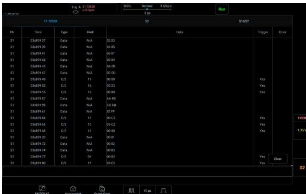
Рисунок 12-33. Текстовый интерфейс 1553B
