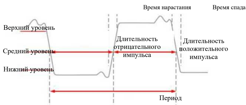
Рисунок 7-4. Временные параметры
