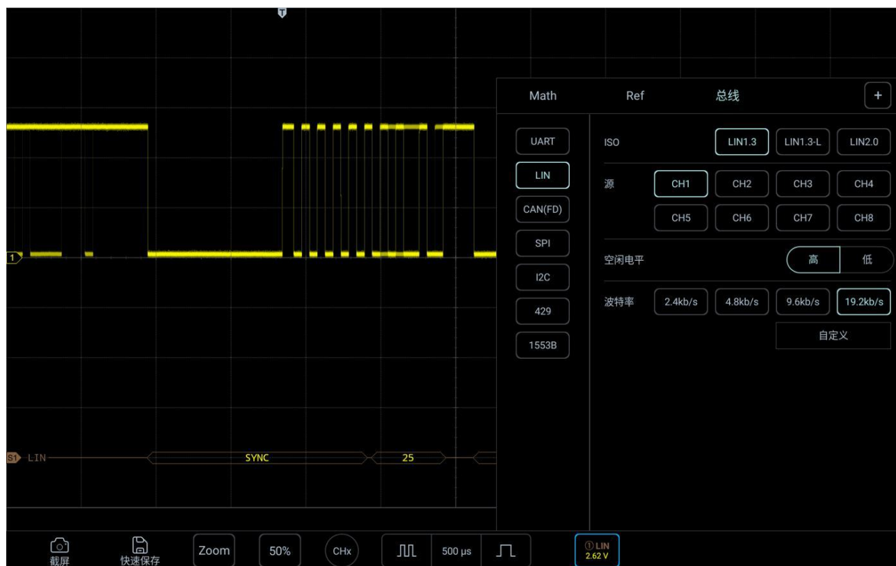
Рисунок 12-10. Меню конфигурации шины LIN
