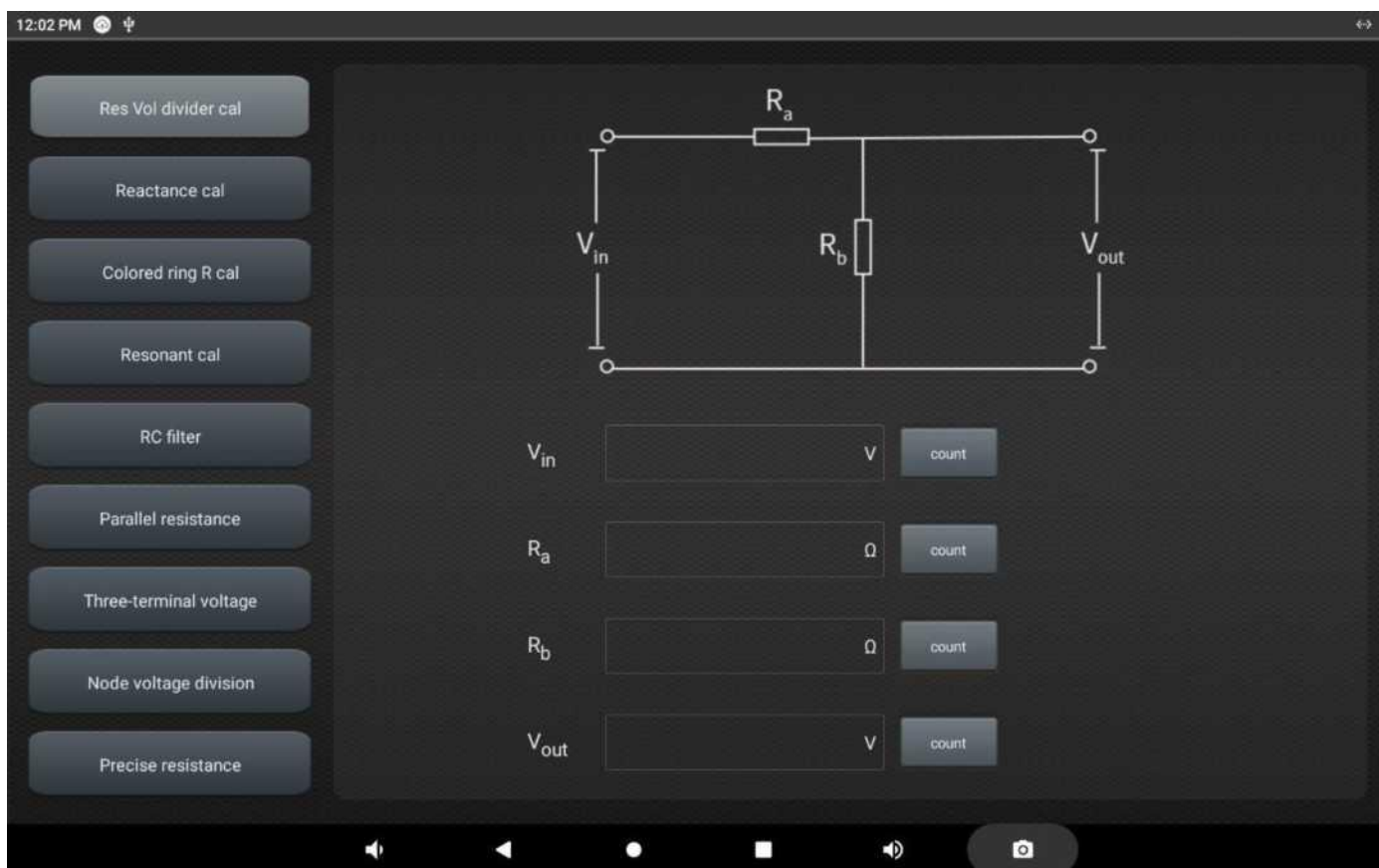
Рисунок 13-10. Функция электронных инструментов для вычисления
