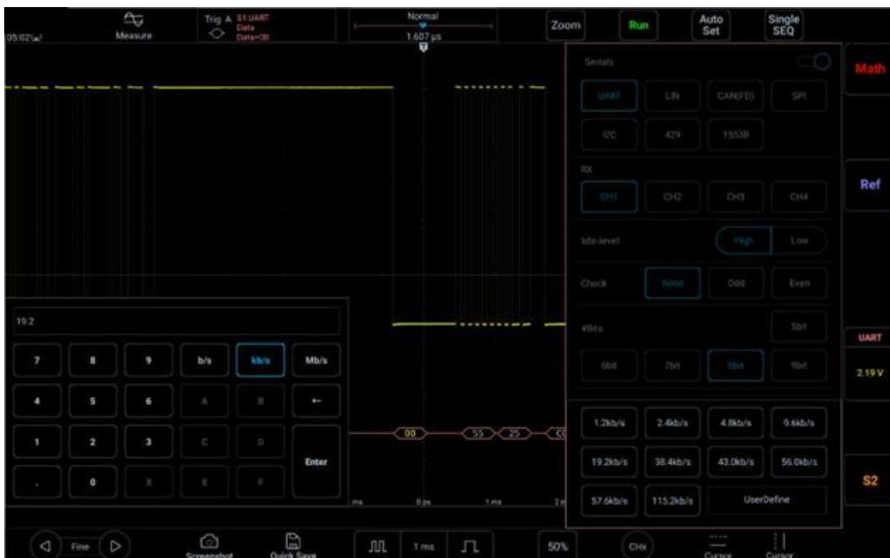
Рисунок 12-5. Настройка скорости передачи данных по умолчанию
