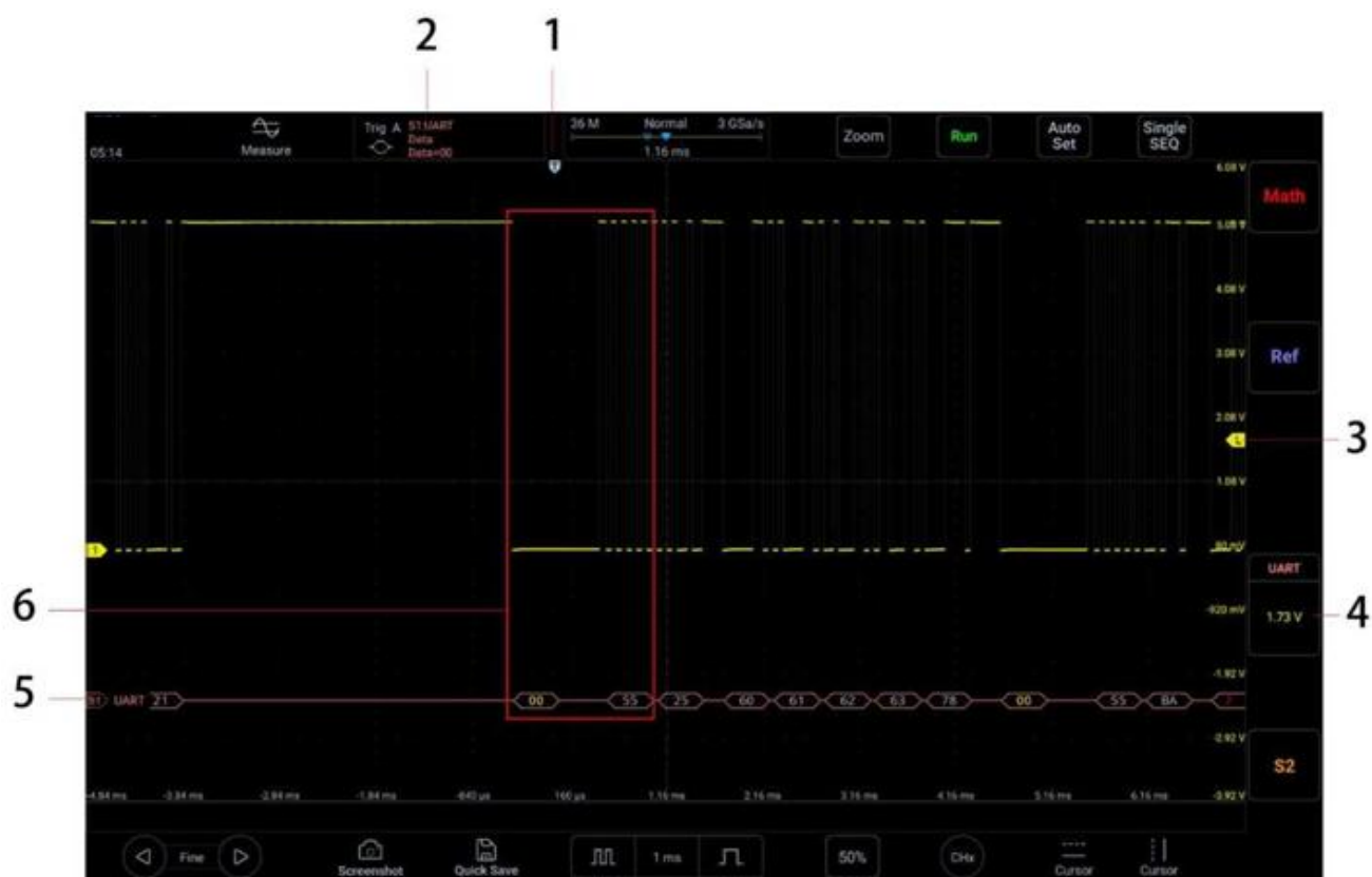
Рисунок 12-8. Графический интерфейс шины UART
