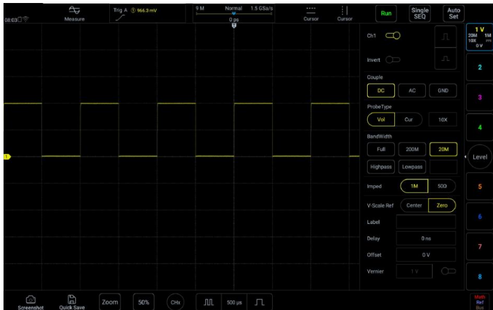
Рисунок 5-12. Полоса пропускания 20М
