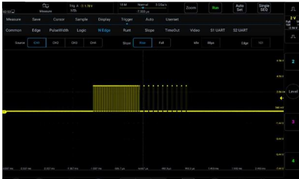
Рисунок 6-23. Меню триггера по N-му фронту
