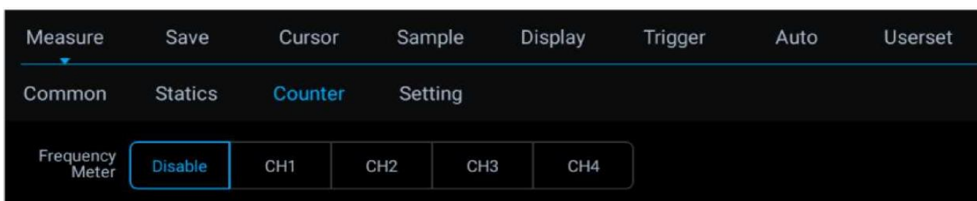
Рисунок 7-14. Открытие меню измерений частотомера
