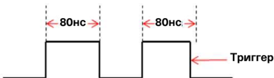
Рисунок 6-16. Время триггера T < 80 нс
