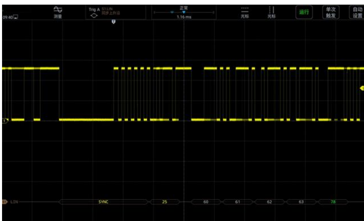
Рисунок 12-12. Графический интерфейс LIN
