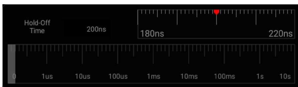
Рисунок 6-11. Интерфейс установки времени удержания триггера
