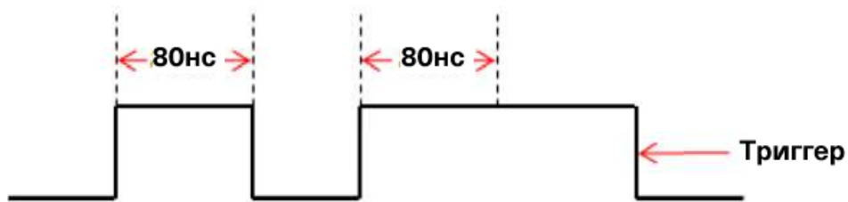
Рисунок 6-17. Время триггера T > 80 нс
