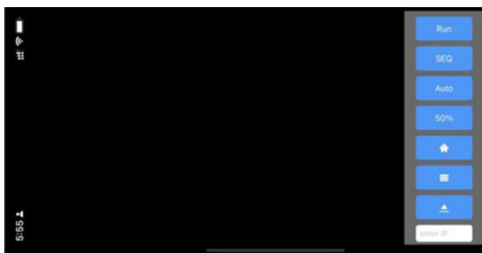
Рисунок 14-6. Интерфейс приложения
