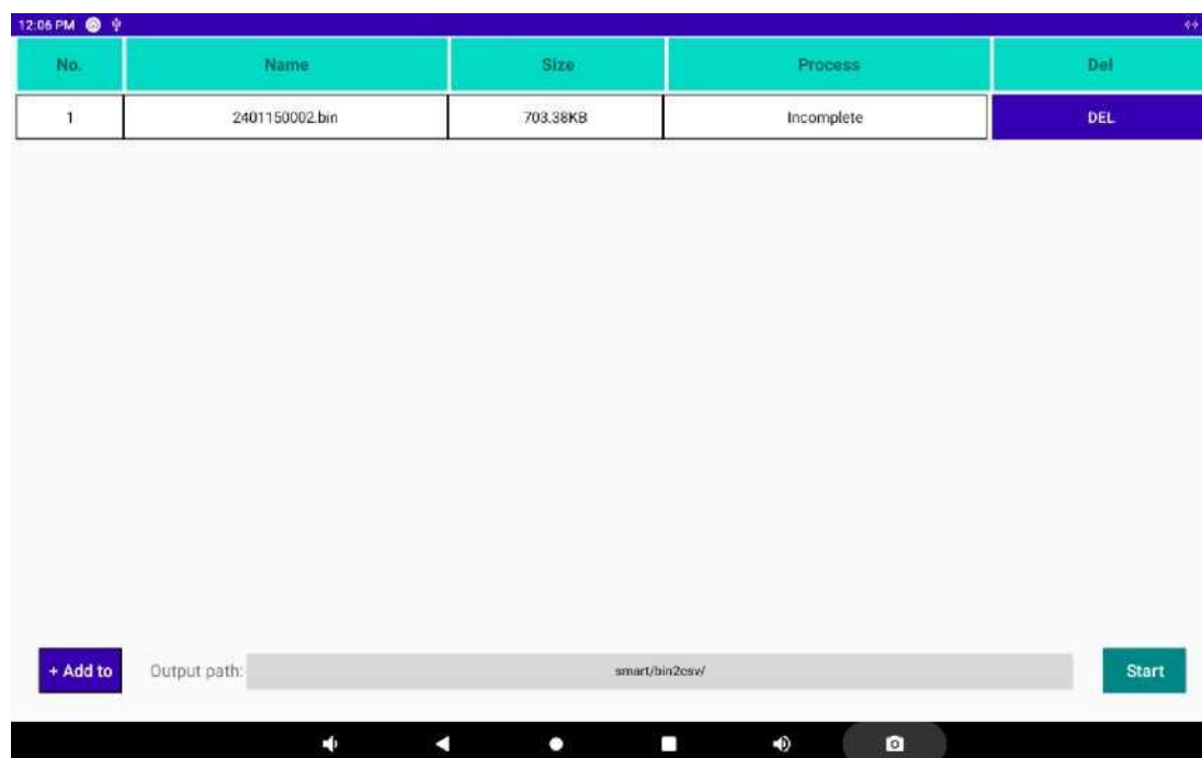
13-17. Приложение BinToCsv
