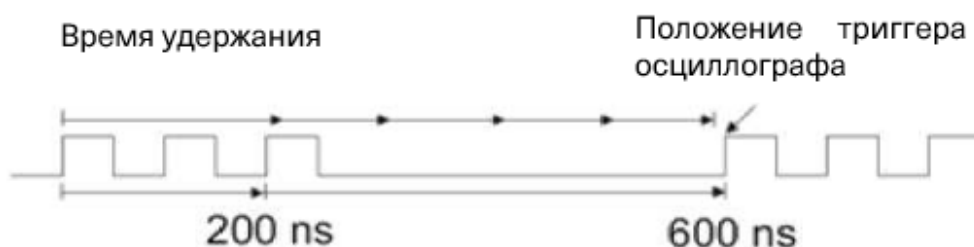
Рисунок 6-10. Время удержания триггера
