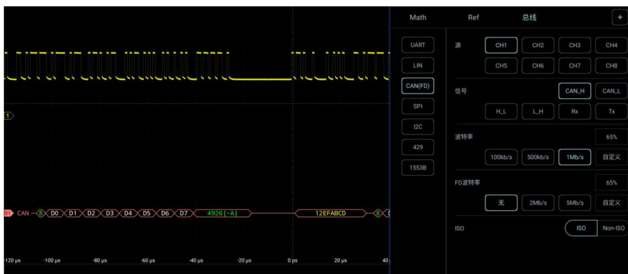
Рисунок 12-14. Меню конфигурации шины CAN/CAN FD
