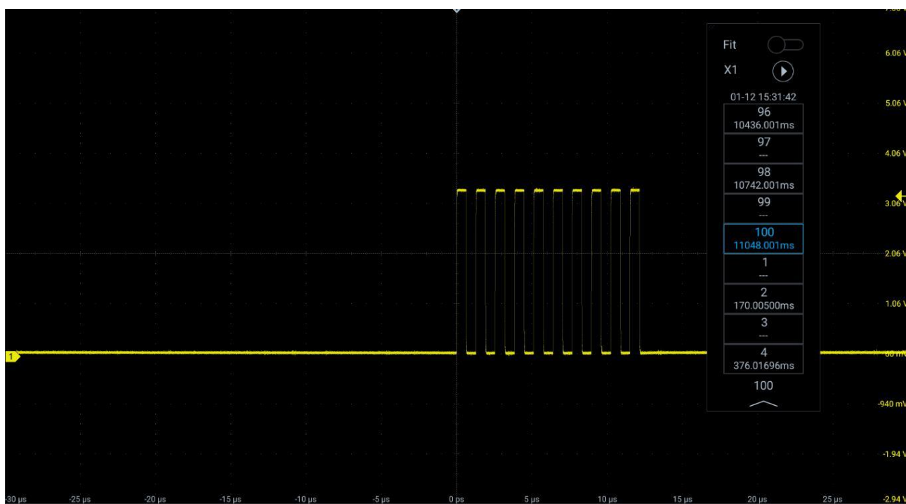
Рисунок 11-12. Сегментированное хранение с просмотром одного кадра
