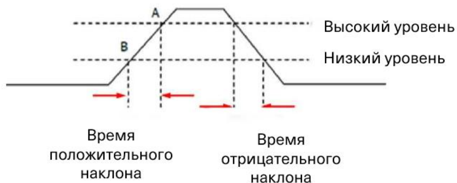
Рисунок 6-26. Время положительного/отрицательного наклона
