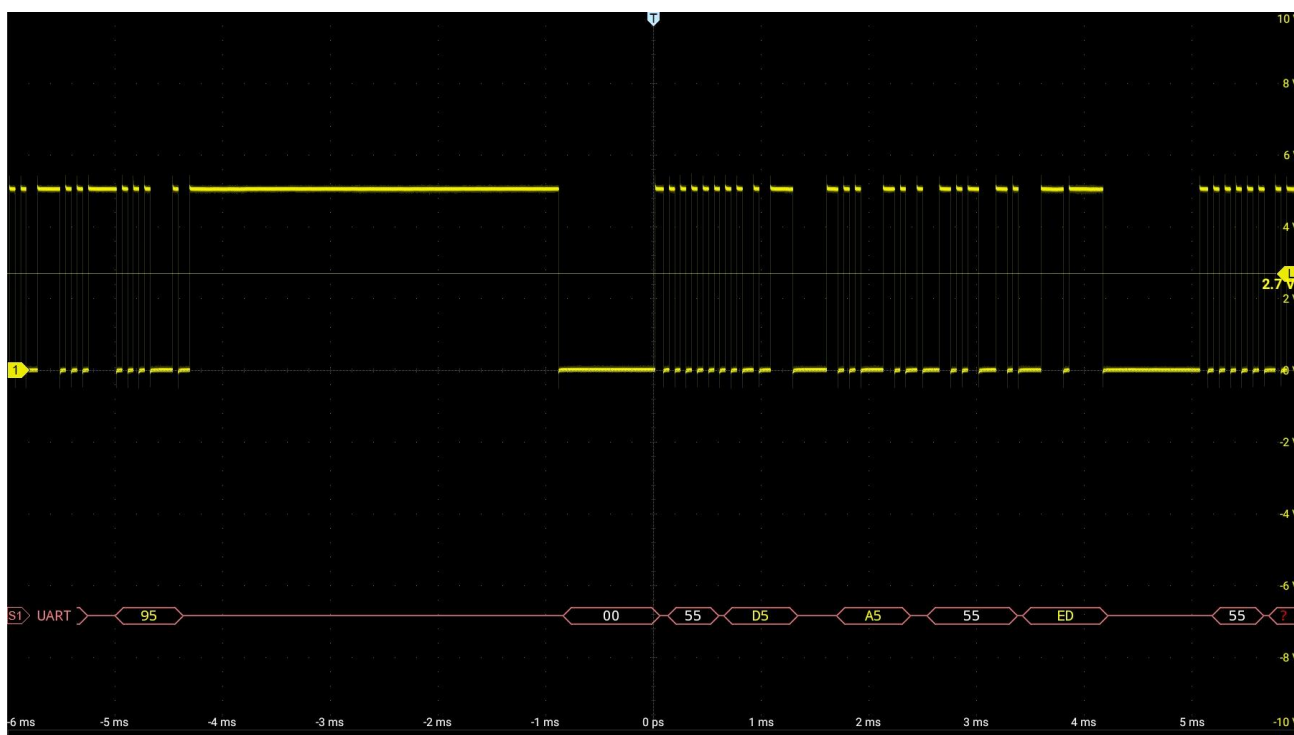
Рисунок 12-7. Регулировка уровня декодирования шины UART
