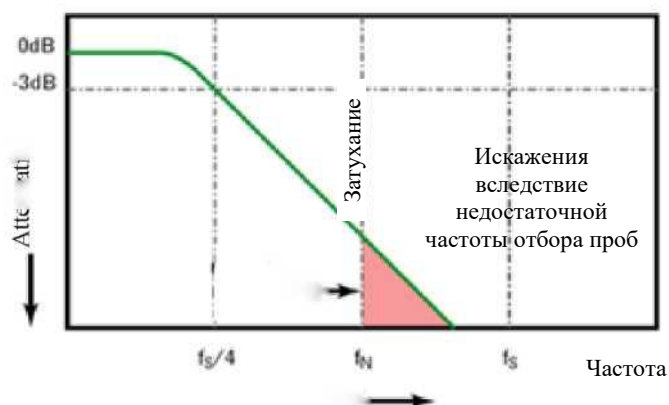
Рисунок 11-3. Частота выборки и полоса пропускания осциллографа
