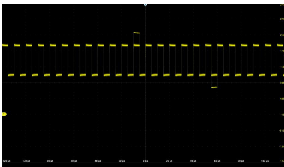
Рисунок 6-3. Аномальный сигнал в периодических сигналах
