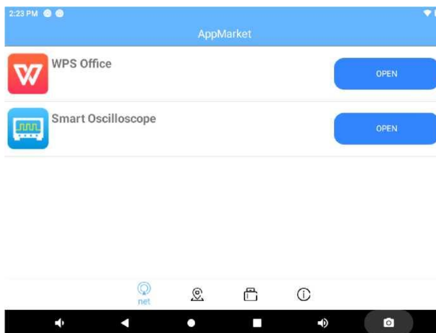
Рисунок 13-2. Магазин приложений
