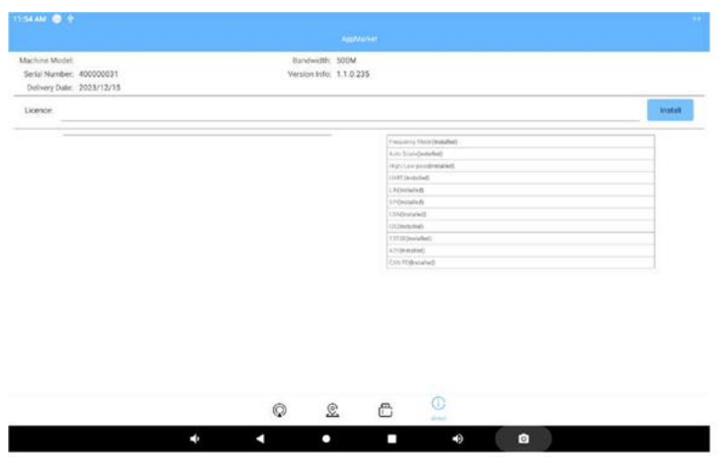
Рисунок 13-3: Интерфейс «About»
