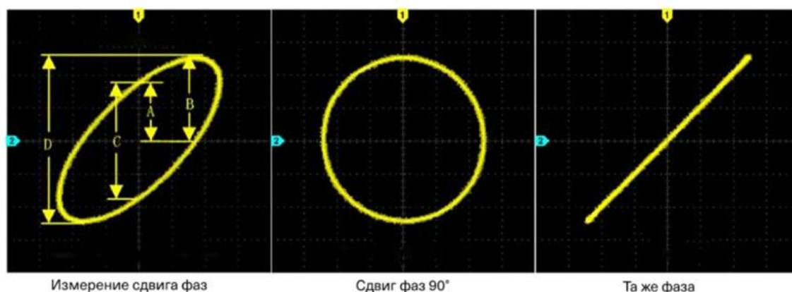
Рисунок 4-8. Сигнал режима строчной развертки XY, центр экрана
