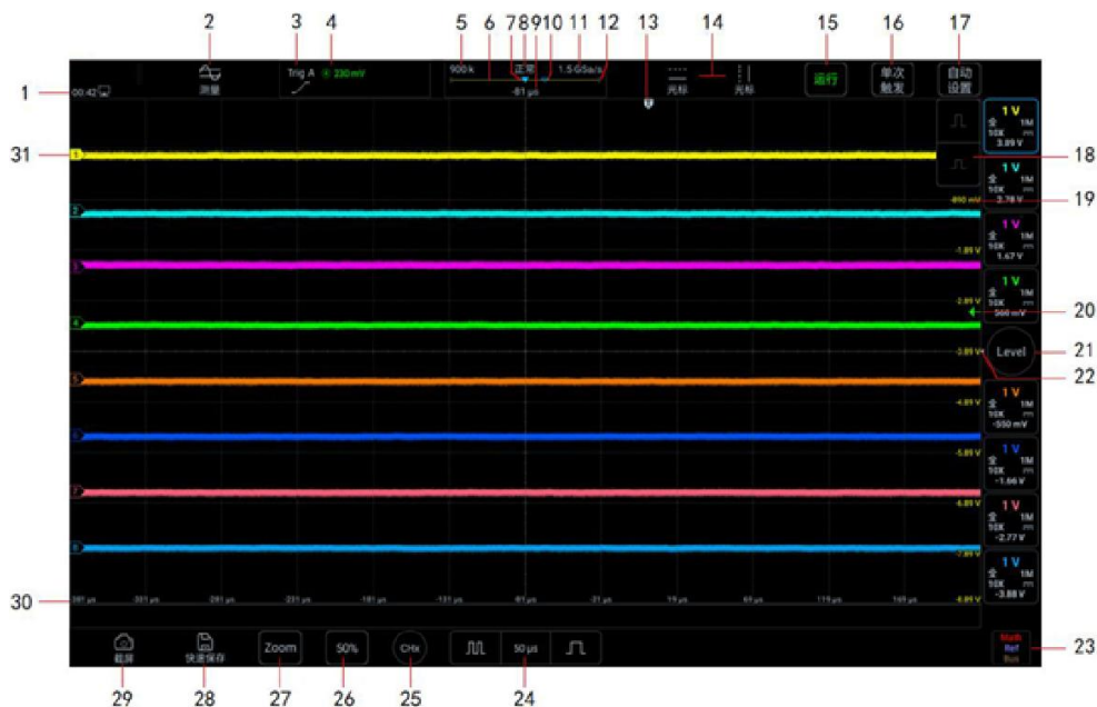
Рисунок 2-4. Отображение интерфейса осциллографа
